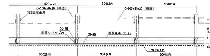
(野縁方向断面図)
