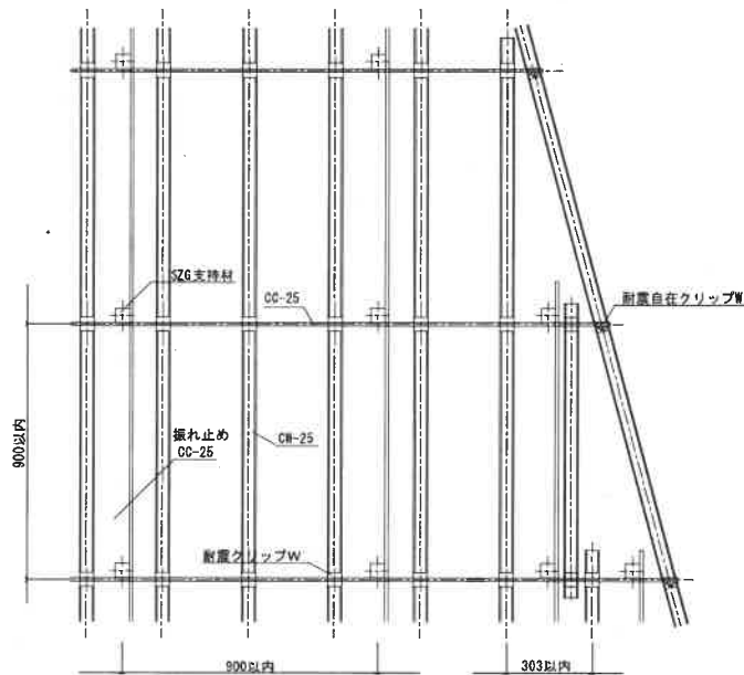
(標準割付図)
