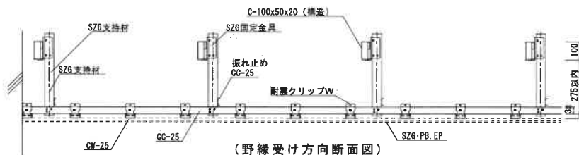
(野縁受け方向断面図)
